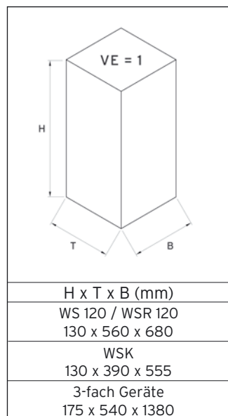
Abb.: Wandgerät WS, 3-fach. Deckel silber, gelb, blau. Art.-Nr.: 1670
