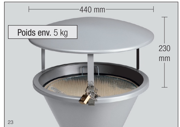
Photo: Toit pour cendrier sablier, revêtement argent, n° d'art. 3318
