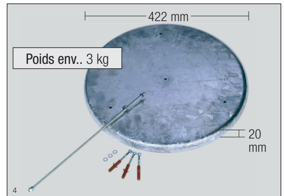
Photo: Ronde de fixation pour cendrier sablier n° d'art. 3320
