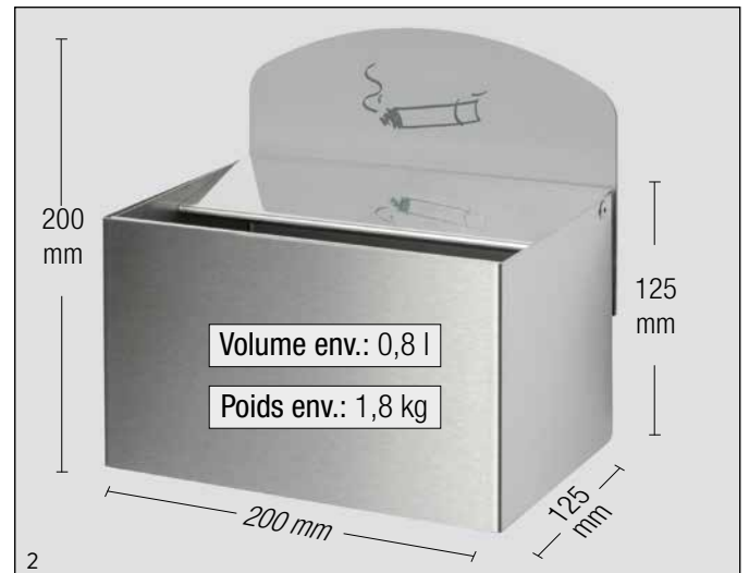
Cendrier mural WH 13, inox, avec panneau. N° d'art.: 14891
