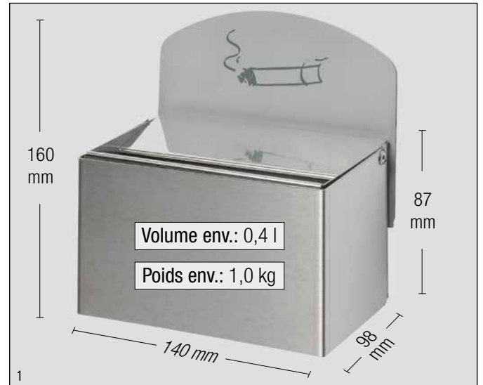
Cendrier mural WH 9, inox, avec panneau. N° d'art.: 14791
