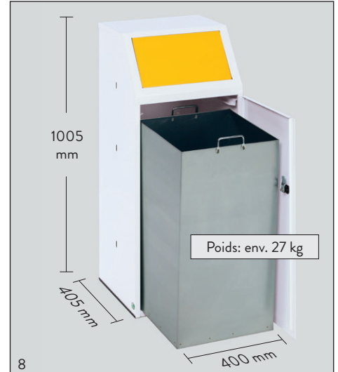
Photo: WSG 69 avec porte en avance, Type B, clapet jaune, n° d'art.: 17161
